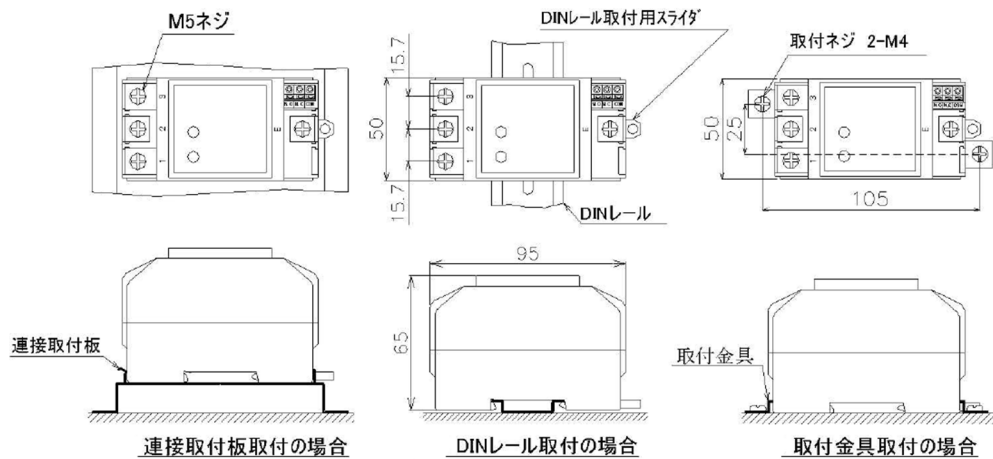
図2 分電盤用 SPD の取付方法
