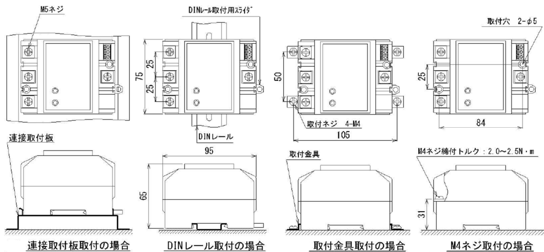
図1 協約寸法 SPD の取付方法
